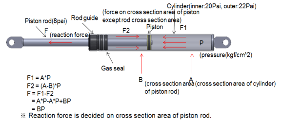
Fig. 9. Piston rod schematic diagram
