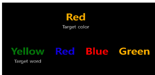
Fig. 1. Stroop task
