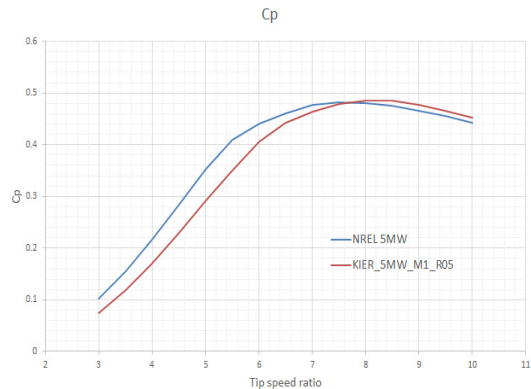
Fig. 9. Blade Cp
