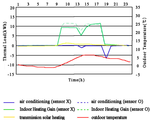
Fig. 11. 2018.1.2 Thermal Load
