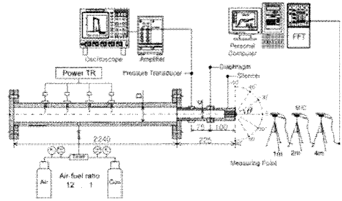
그림 1. 충격성 소음 발생기 개략도 및 측정 장치 구성도
