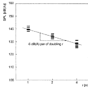
그림 4. 소음 발생기로부터 방사된 충격성 소음의 거리감쇠 특성
