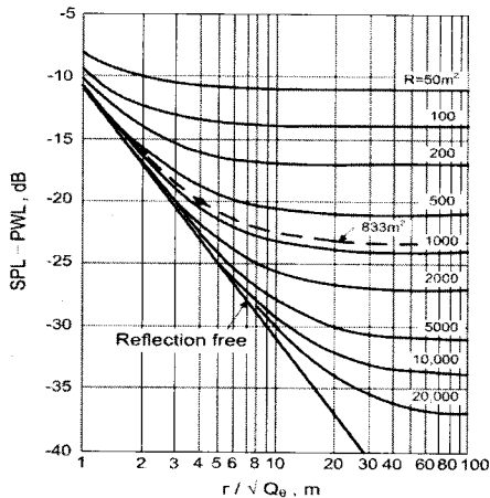
그림 2. 실정수 R에 따른 거리별 음압레벨과 음향 파워레벨의 관계
