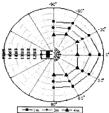
그림 3. 소음 발생기로부터 방사된 충격성 소음의 거리별 지향성 비교
