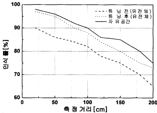
[그림 7] 거리에 따른 RFID 인식을 측정 결과
