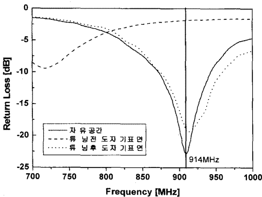
[그림 4] 제작된 안테나의 S11 측정 결과
