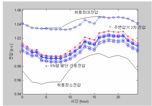
[그림 10] 그림9와 같은 DG연계시스템에 자율분산협조제어 알고리즘을 적용한 경우의 전압특성곡선
