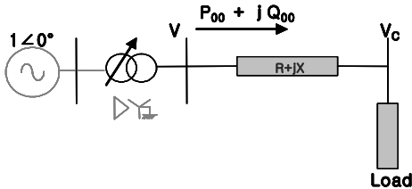
[그림 1] 단일상가부하로 표현된 배전계통모델
