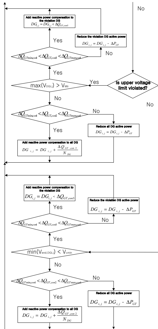
[그림 6] 자율분산협제어 알고리즘
