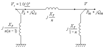
[그림 3] 주변압기의 등가회로
