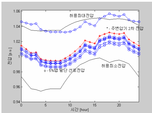
[그림 9] DG연계후 전압특성곡선
