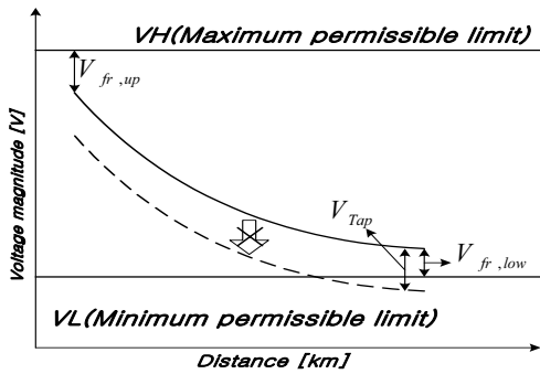
(b) ULTC동작시 전압조정범위를 벗어나는 경우
