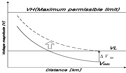
(b) DG연계되지 않은 선로가 저전압으로 되는 경우
