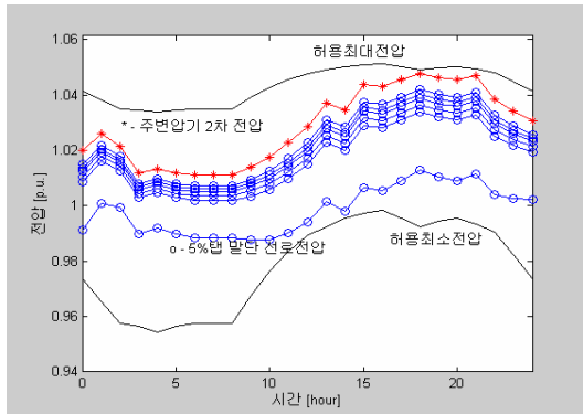
[그림 8] DG연계되지 않은 경우 전압특성곡선
