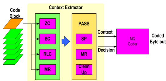
[그림 3] Context 추출기의 Flowchart.
