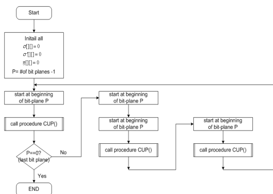
[그림 2] BPC 알고리즘 FlowChart.
