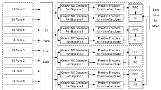
[그림 4] 제안한 EBCOT의 Top Module.
