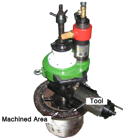
[그림 9] 선삭 가우징 실험 장치
