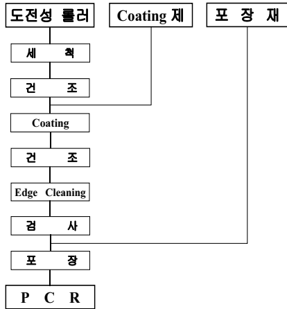
[그림 5] 대전 롤러의 제조 공정
