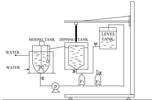
[그림 8] 코팅 장치의 전체적인 구성도
