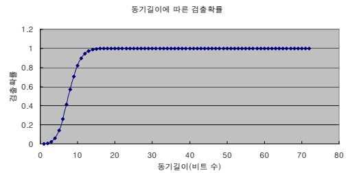
[그림 8] 동기 길이 대비 검출확률
