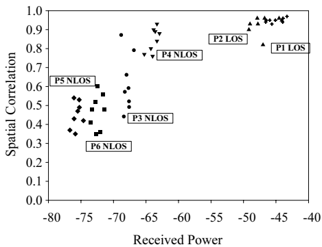
[그림 7] 수신파위에 따른 공간 상관 계수
