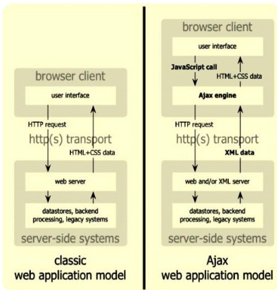
[그림 2] 전통적인 웹어플리케이션 모델과 AJAX 웹어플리케이션 모델 비교
