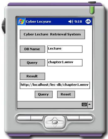
[그림 8] ADO.NET을 이용한 PDA에서의 non-XML 데이터 검색 구현
