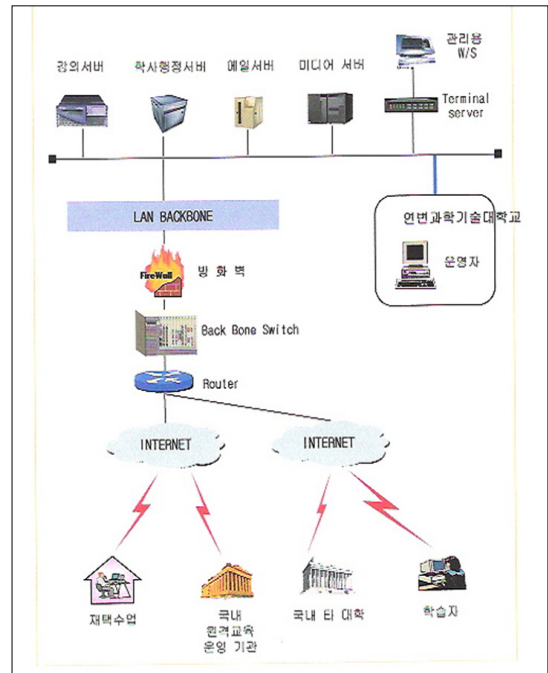
[그림 3] E-Learning 물리적 시스템 구성도
