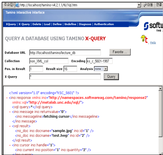
[그림 7] X-Query를 이용한 검색 결과
