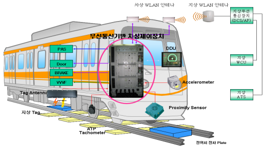
[그림 2] 무선통신기반 차상제어장치의 구성도
