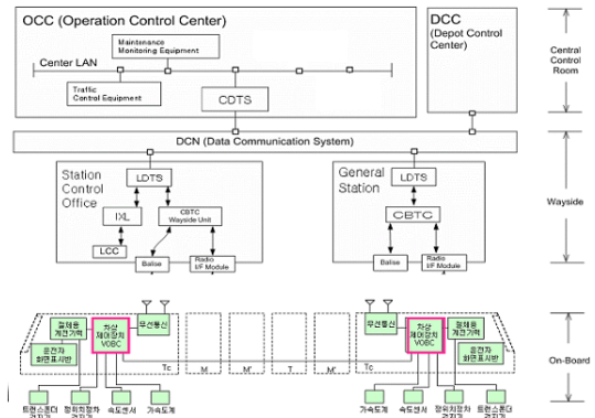
[그림 1] 무선통신기반 열차제어시스템의 구성도
