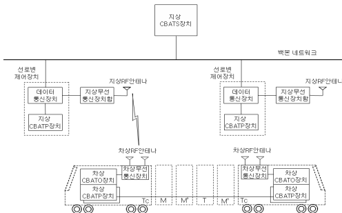
[그림 3] 차상제어장치와 지상장치의 인터페이스
