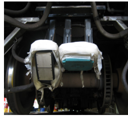
도플러/Proximity 센서
