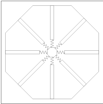
[그림 3] 8-way 저항성 전력 분배기 회로
