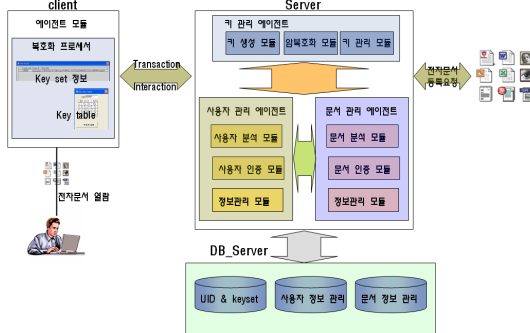
[그림 4] 제안하는 시스템 구조
