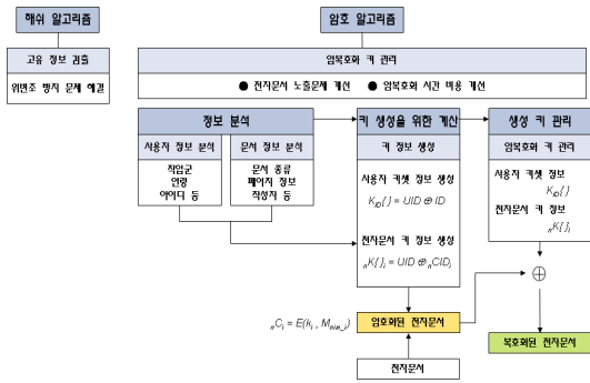
[그림 5] 제안기법의 프로세스 흐름도
