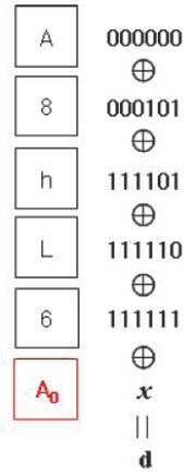
[그림 10] 마지막 행값 생성 과정
