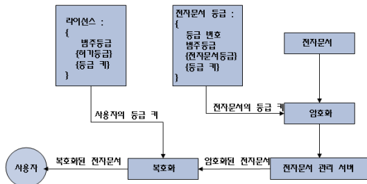
[그림 3] 전자문서의 암호화와 복호화
