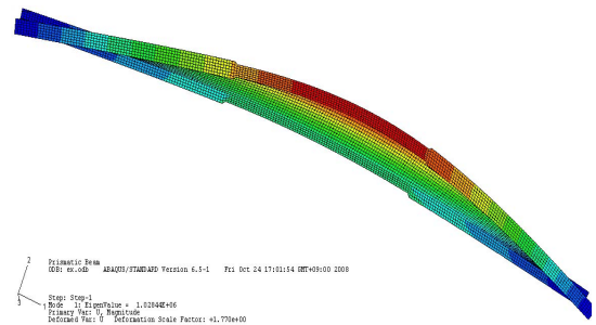
[그림 4] 좌굴 모드 ( \rho=0.3 )
