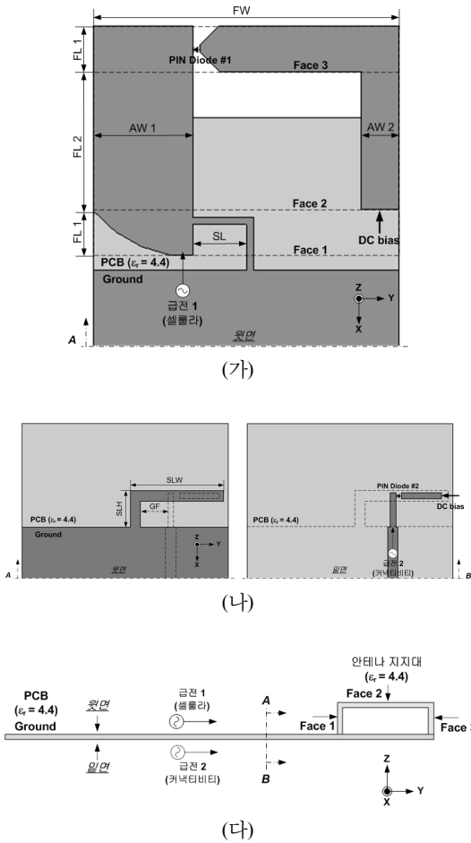
[그림 2] 제안된 안테나의 구성도 (가) 셀룰러 대역용 주파수 재구성 안테나 (전개도), (나) 커넥티비티 대역용 주파수 재구성 안테나, (다) PCB 상 두 안테나의 측면도
