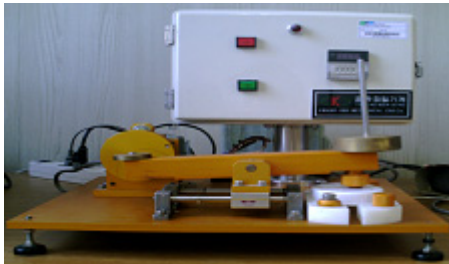
[그림 2] 내마모 테스트 평가방법
