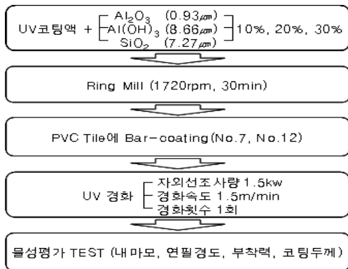
[그림 1] 코팅액 제조 및 UV경화 코팅조건
