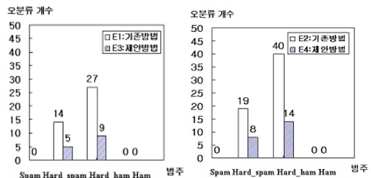
(a) 학습오류 0% (b) 학습오류 10%
