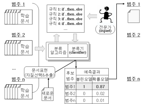
[그림 2] 자동문서분류시스템의 기본 개요
