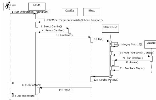
[그림 4] ETOM + RPost 시스템 설계를 위한 클래스 다이어그램과 시퀀스 다이어그램
