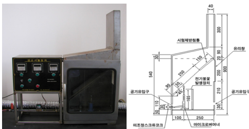
[그림 4] 연소시험장치
