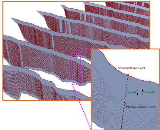
[그림 4b] ADCP의 2차원과 3차원 측정 자료가 기존의 1차원 하천망도와 연계되는 과정 ([12])
