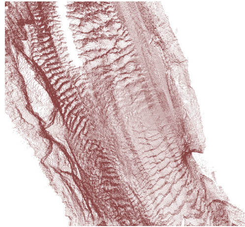
(b) 복수빔 음파수심계로 측정된 하상 자료
