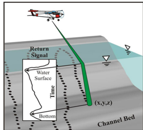
[그림 3] 공중 전파수심계의 개념도
