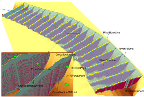
[그림 5] Arc River 자료 모델에 기반하여 저장된 ADCP 자료
