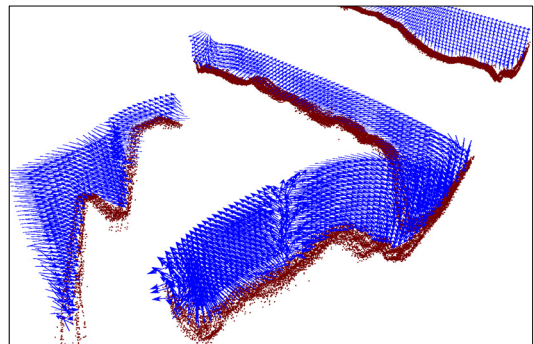
[그림 1] 선박에 탑재된 ADCP를 통해 측정된 유속분포 및 하상 자료
