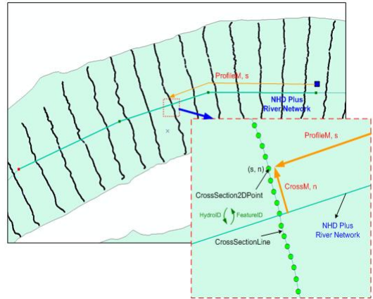
[그림 4a] ADCP의 2차원과 3차원 측정 자료가 기존의 1차원 하천망도와 연계되는 과정 ([12])
