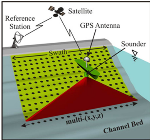
(a) 선박에 탑재되어 광폭의 하상을 측정하는 방식인 복수빔 음파수심계의 개념도
