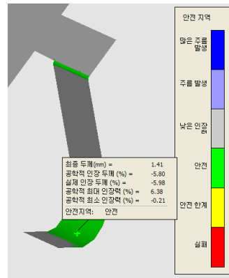
[그림 7] 3차 벤딩 안전지역분석결과 [Fig. 7] 3rd bending safety area analysis
