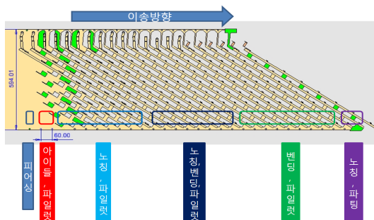
[그림 1] 터미널 UV 단자의 스트립 레이아웃도 [Fig. 1] Terminal strip layout drawing
