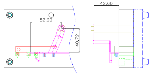
[그림 19] 구멍간 위치수정 [Fig. 19] Modify the hole between the position
