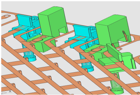
[그림 10] 벤딩 펀치 및 다이블록 설계 [Fig. 10] Bending punch and the die block design
