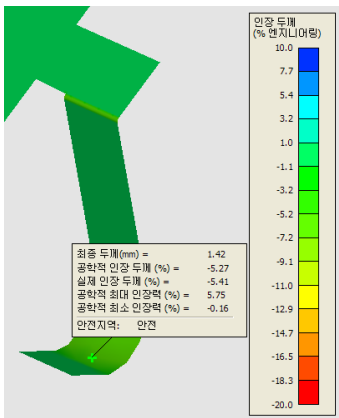
[그림 6] 3차 벤딩 인장두께분석결과 [Fig. 6] Thickness of the third bending tensile analysis
