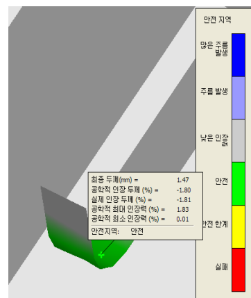
[그림 3] 1차 벤딩 안전지역분석결과
