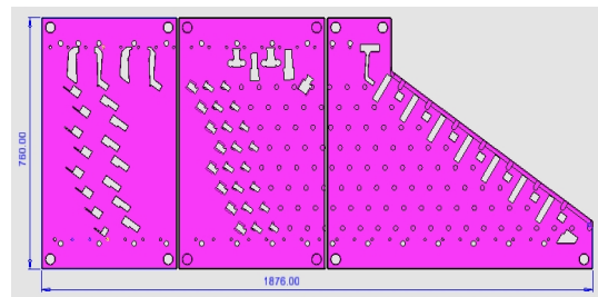
[그림 8] 다이 플레이트 [Fig. 8] Die Plate
