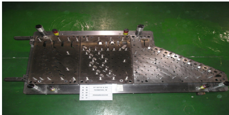
[그림 15] 하형 조립 [Fig. 15] Under Assembly
