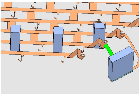
[그림 11] 파팅 펀치 설계 [Fig. 11] Parting Punch Design
