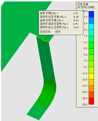
[그림 4] 2차 벤딩 인장두께분석결과 [Fig. 4] Thickness of the secondary bending tensile analysis
