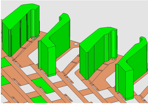
[그림 9] 노칭 펀치 설계 [Fig. 9] Notching Punch Design
