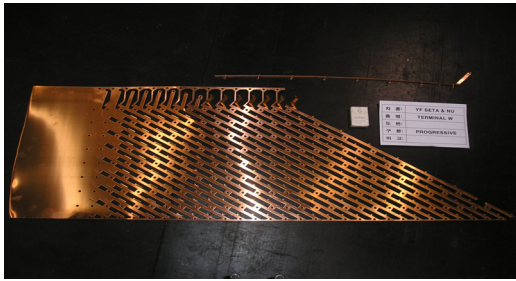
[그림 20] 최종완성된 스트립 [Fig. 20] Final finished strip
