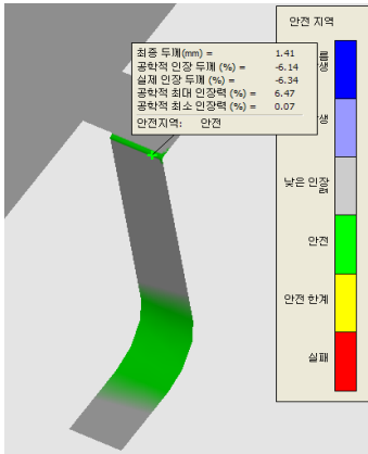
[그림 5] 2차 벤딩 안전지역분석결과 [Fig. 5] 2nd bending safety area analysis
