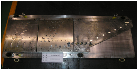
[그림 14] 상형 조립 [Fig. 14] Up Assembly
