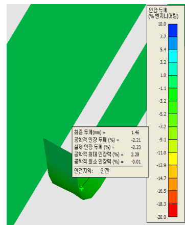
[그림 2] 1차 벤딩 인장두께분석결과
