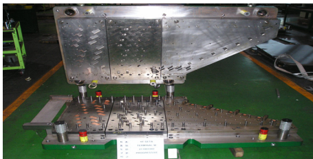
[그림 16] 전체 조립 [Fig. 16] Entire assembly
