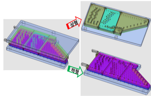
[그림 12] 상,하형 조립도 [Fig. 12] entire assembly drawings
