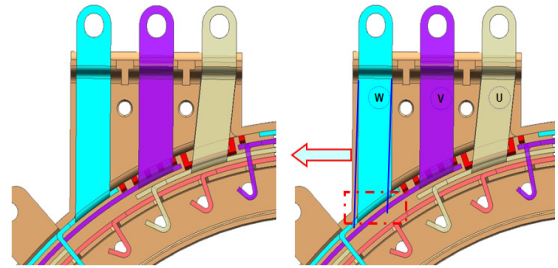
[그림 17] 단자부 벤딩라인 수정 [Fig. 17] Minor modifications bend the line terminals
