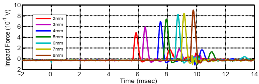
[그림 4] 인가전압과 간격별 솔레노이드 충격력 [Fig. 4] The supply voltage and the impact force of solenoid at the some different gaps
