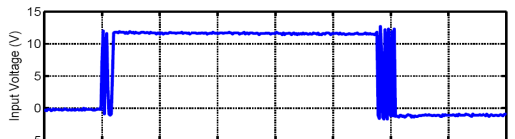
[그림 3] 솔레노이드 인가 전압 [Fig. 3] The supply voltage to solenoid
