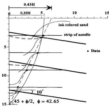
(b) 파괴모드 (네일길이=12cm, 설치각=10°)
