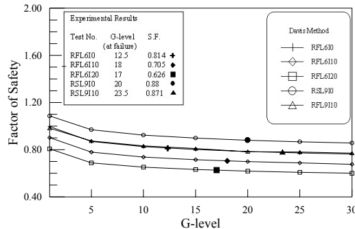
[그림 21] Davis 방법에 의한 안전율 산정
