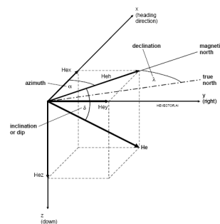
[그림 2] 지구 자기장 벡터
