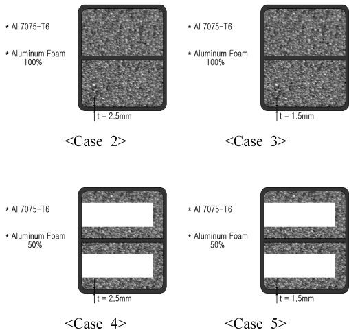
[그림 4] 알루미늄 폼과 범퍼 폼의 조립형상
