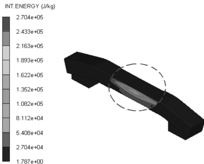
【그림 10】 Case 2의 변형량 및 내부에너지
