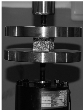
[그림 5] 기본 물성 테스트 사진
