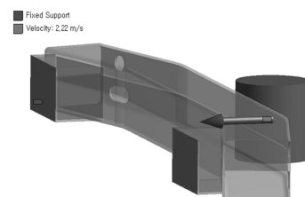
[그림 8] 구속 및 속도 조건
