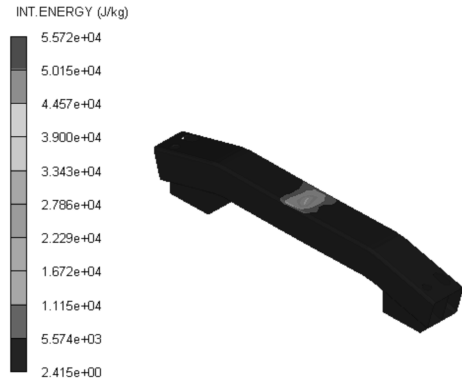
【그림 9】 Case 1의 변형량 및 내부에너지
