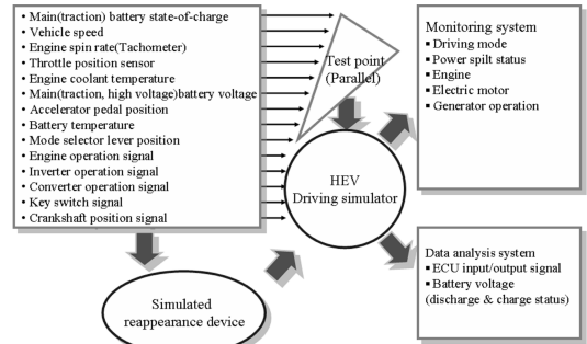
[그림 1] THS의 구성과 제어 범위
