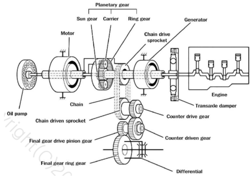
【그림 3】 동력분할장치와 기어 트레인의 구성
