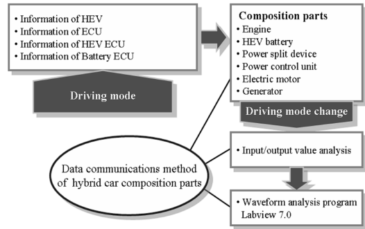
[그림 5] 하이브리드 시스템의 데이터 입출력
