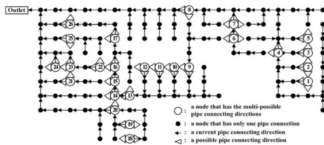
(a) 현재 우수관망 개략도
