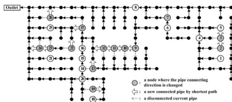
(c) 최적 우수관망 개략도
