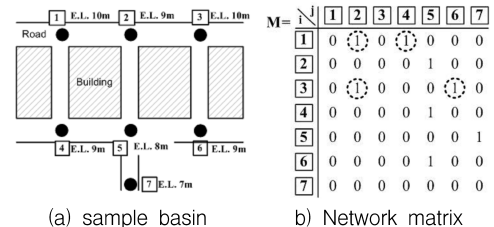
[그림 2] 도시구역 network matrix(이정호, 2010)[1]
