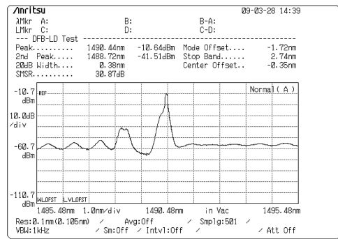
[그림 9] 개선되어 확인된 SMSR 시험결과
