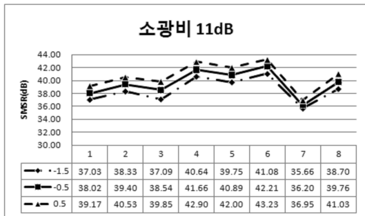
[그림 8] 소광비 11 dB 고정 후, 광 파워 출력 변화에 따른 SMSR 시험결과
