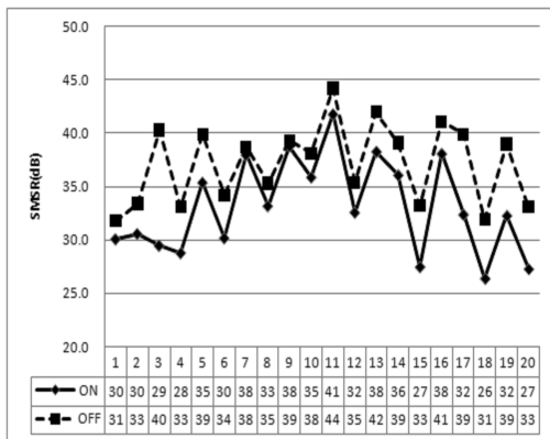
[그림 2] 변조 유무에 따른 시험결과 (점선: 무변조 상태, 실선: 변조 상태)
