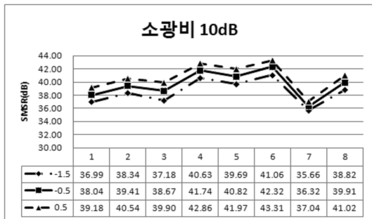
[그림 7] 소광비 10 dB 고정 후, 광 파워 출력 변화에 따른 SMSR 시험결과
