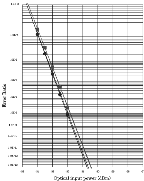
[그림 10] 광수신기의 개선된 수신감도 BER 커브
