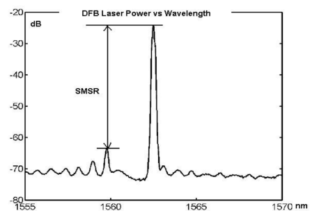
[그림 1] SMSR 개요[3]
