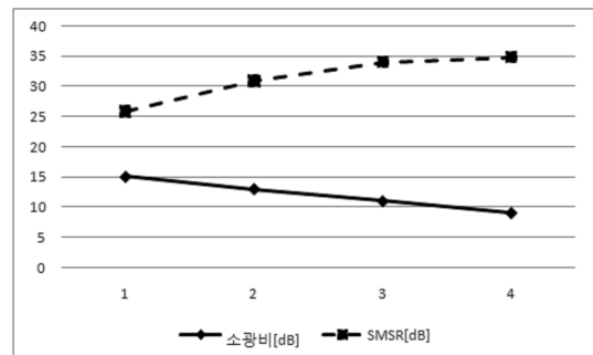
[그림 3] 1.25 Gbps에서의 소광비 변화에 따른 SMSR 시험결과
