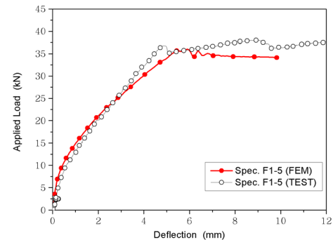
[그림 11] 실험체 F1-5의 하중-변위 곡선 [Fig. 11] Load-displacement curves for F1-5
