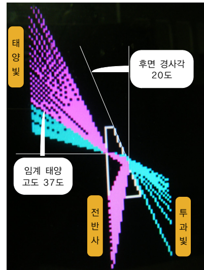
[그림 6] 후면 경사각 20°에 대한 태양고도 변화와 전반사 시뮬레이션
