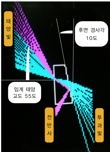
[그림 4] 후면 경사각 10°에 대한 태양고도 변화와 전반사 시뮬레이션
