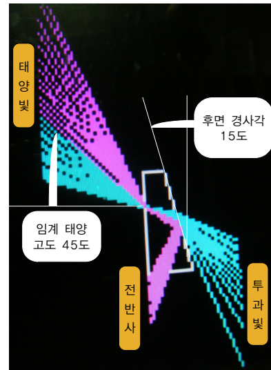
[그림 5] 후면 경사각 15°에 대한 태양고도 변화와 전반사 시뮬레이션
