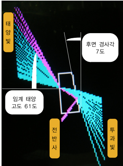
[그림 3] 후면 경사각 7°에 대한 태양고도 변화와 전반사 시뮬레이션
