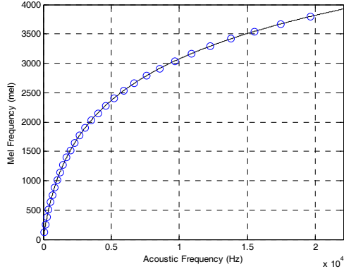
[그림 8] 삼각 Mel-weighted Filter Bank의 중간 주파수(원의 각 중심은 각 필터의 중간 주파수에 상응함) [Fig. 8] Mid frequencies of the Triangular Mel-weighted Filter Bank (each center of circle corresponds to mid frequency of each filter)
