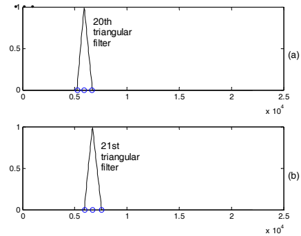
[그림 9] 각 삼각 필터의 제작 [Fig. 9] An illustration of establishing each triangular filter
