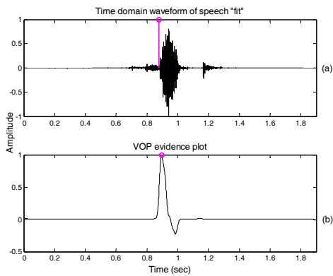
[그림 14] VOP 증거 plot
