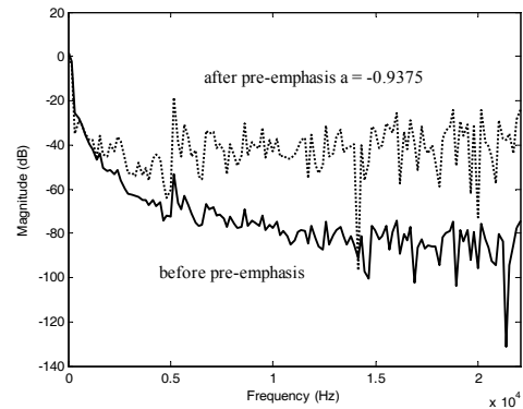
[그림 3] 프리엠퍼시스 전후의 말 신호의 주파수 응답(점선은 평평하게 된 음성 스펙트럼)
