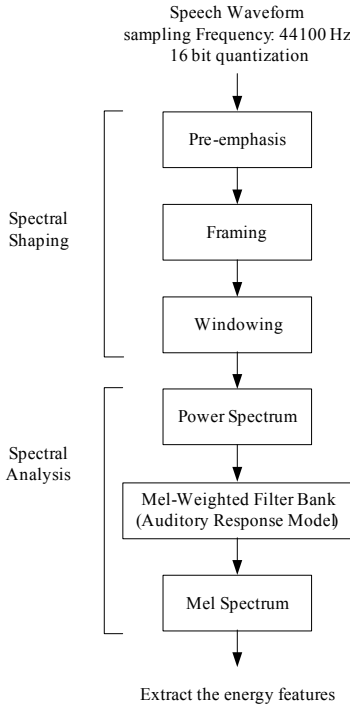
[그림 2] 특징 추출 흐름
