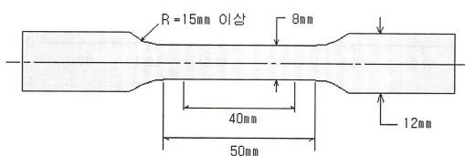
[그림 2] 인장시험편 형상
