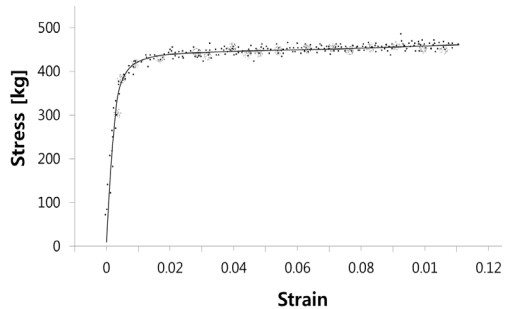
[그림 4] 진응력-진변형률 선도
