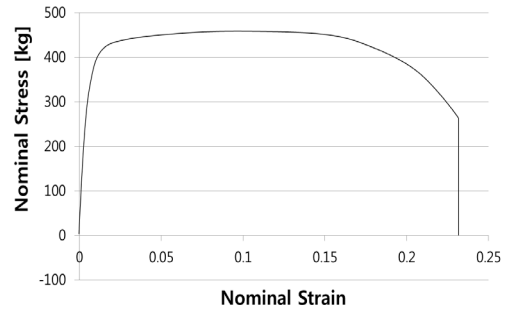
[그림 3] 공칭응력-공칭변형률 선도
