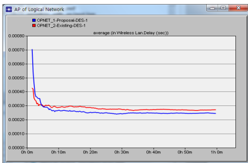
[그림 10] AP 노드 비교 분석 (Delay) [Fig 10] AP Node Statistic Compare (Delay)
