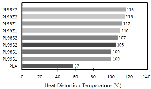
[그림 2] PLA 컴파운드의 열변형 온도
