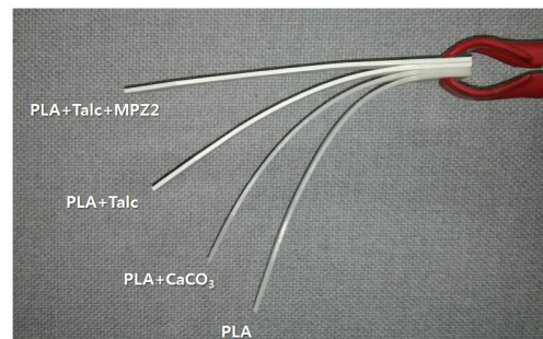
[그림 3] PLA 컴파운드의 내열성 테스트
