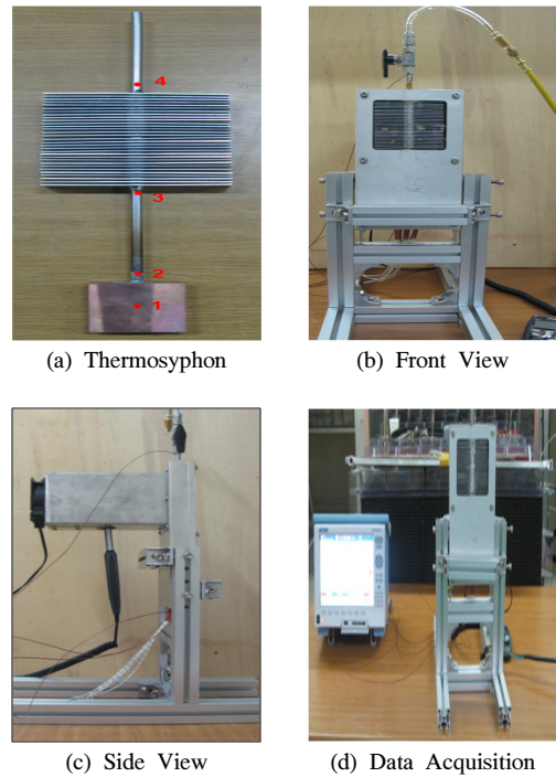
[그림 1] 써모사이폰 실험장치 사진
