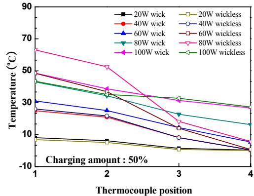
[그림 6] 심지 유무에 따른 써모사이폰의 온도 특성 비교 실험장치 개략도(0℃/50%)
