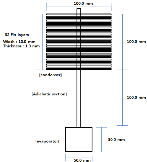
[그림 2] 개발된 써모사이폰의 개략도
