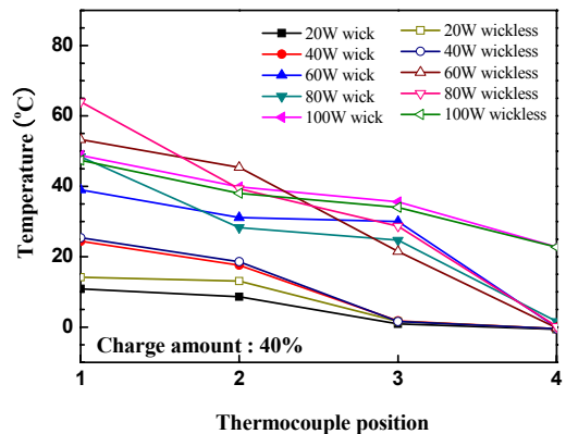
[그림 4] 심지 유무에 따른 써모사이폰의 온도 특성 비교 실험장치 개략도(-20°C/40%)
