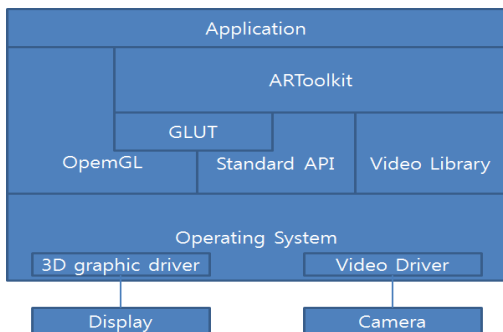
[그림 3] ARToolkit의 구조
