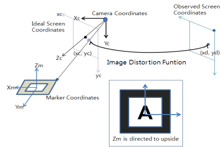
[그림 4] 카메라와 마커간의 좌표계
