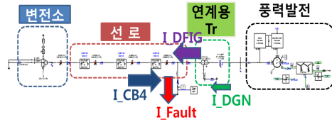
[그림 17] 1선지락전류 수집지점(Case 3) [Fig. 17] Collection points of a single line ground faults current(Case 3)
