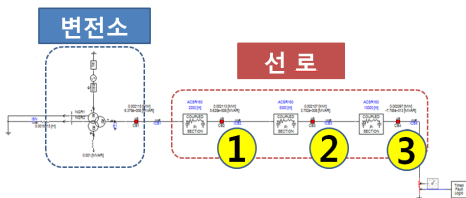
[그림 8] Case 1 시뮬레이션의 구성도 [Fig. 8] Simulation configuration of case 1
