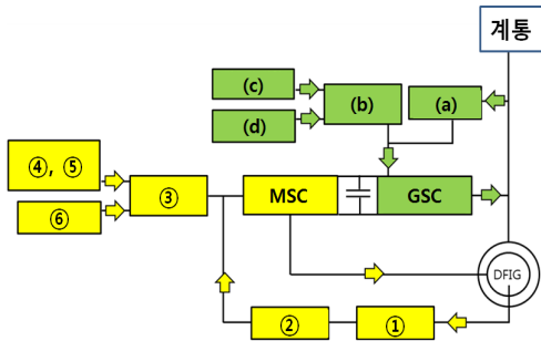
[그림 5] DFIG의 제어블록도 [Fig. 5] Control block of DFIG
