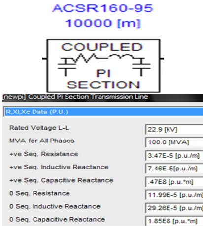
[그림 4] 배전선로 ACSR160모델과 내부변수 값 [Fig. 4] Model and internal value of ACSR160
