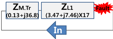
[그림 12] 정상분 % 임피던스 맵(Case 2) [Fig. 12] Positive phase sequence component of equivalent circuit(Case 2)
