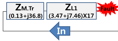
[그림 9] 정상분 % 임피던스 맵(Case 1) [Fig. 9] Positive phase sequence component of equivalent circuit(Case 1)
