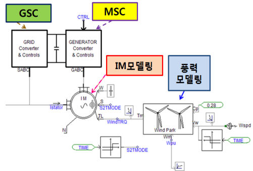
[그림 6] DFIG 모델링 [Fig. 6] Modeling of DFIG
