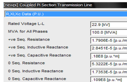
[그림 3] 배전선로 CNCV 325모델과 내부변수 값
