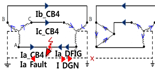
배전용변전소 배전선로 연계용 Tr DFIG [그림 19] Case 3의 1선지락전류 분석 [Fig. 19] Analysis for a single line ground faults current (Case 3)
