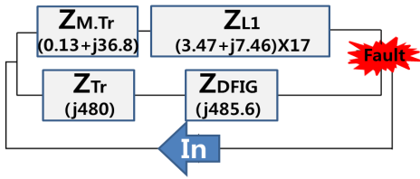
[그림 15] 정상분 % 임피던스 맵(Case 3) [Fig. 15] Positive phase sequence component of equivalent circuit(Case 3)
