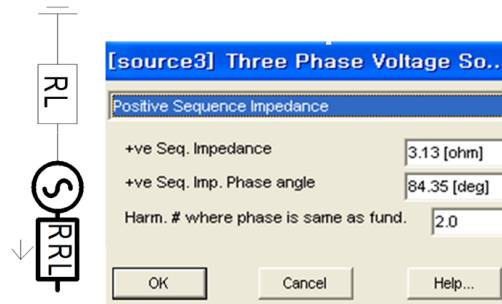
[그림 2] 154kV 전원계통 모델과 내부변수 값
