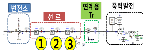
[그림 7] 모델 배전계통 [Fig. 7] Model distribution network
