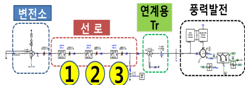
[그림 14] Case 3의 시뮬레이션 구성도 [Fig. 14] Simulation configuration of case 3
