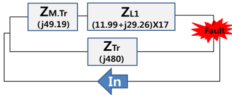
[그림 16] 영상분 % 임피던스 맵(Case 3) [Fig. 16] Negative phase sequence component of equivalent circuit(Case 3)
