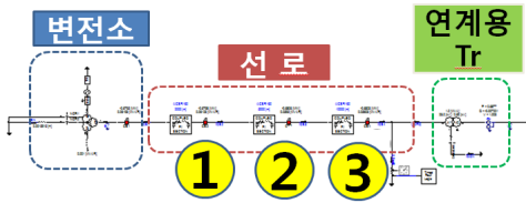
[그림 11] Case 2 시뮬레이션의 구성도 [Fig. 11] Simulation configuration of case 2
