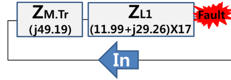
[그림 10] 영상분 % 임피던스 맵(Case 1) [Fig. 10] Negative phase sequence component of equivalent circuit(Case 1)
