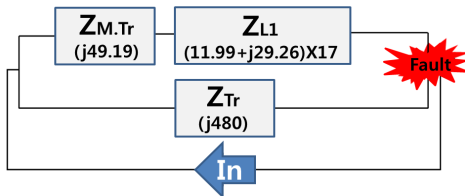
[그림 13] 영상분 % 임피던스 맵(Case 2) [Fig. 13] Negative phase sequence component of equivalent circuit(Case 2)
