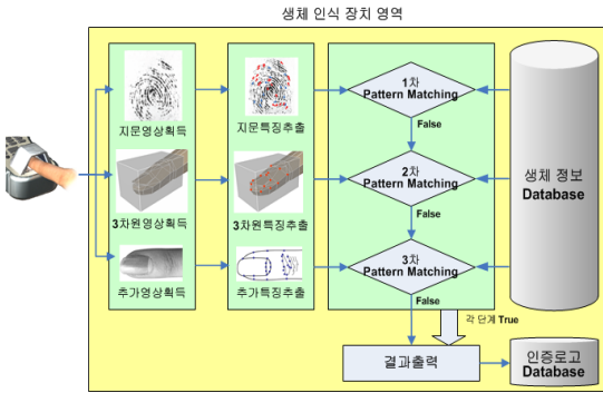
[그림 15] 독립형태 시스템 구성도 [Fig. 15] System configuration of standalone type
