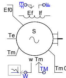
[그림 8] PSCAD/EMTDC에 의한 DG모델링 [Fig. 8] DG Modeling By PSCAD/EMTDC
