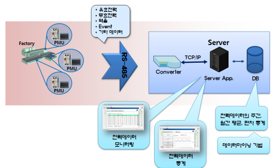
[그림 2] 전력에너지 관리 시스템 [Fig. 2] Electronic-Power Management System
