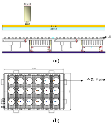
[그림 6] (a) 휘도 측정 모듈 (b) 측정 위치
