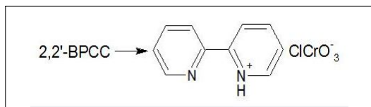
[그림 2] 2,2'-비피리딘늄 클로로크로메이트 [C 10 H 8 N 2 HCrO 3 Cl] [Fig. 2] 2,2'-bipyridinium chlorochromate [C 10 H 8 N 2 HCrO 3 Cl]
