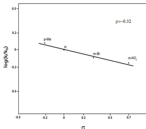
[그림 6] 2,2'- 비피리딘늄 클로로크로메이트에 의한 치환 벤질 알코올류의 산화반응에서 하메트 도시, 303K
