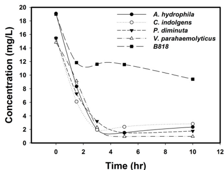
[그림 4] 선별된 균주별 암모니아성 질소 제거효율.
