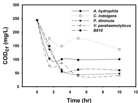
[그림 3] 선별된 균주별 유기물 제거효율.
