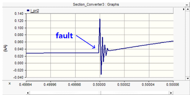
(b) 사고전류
