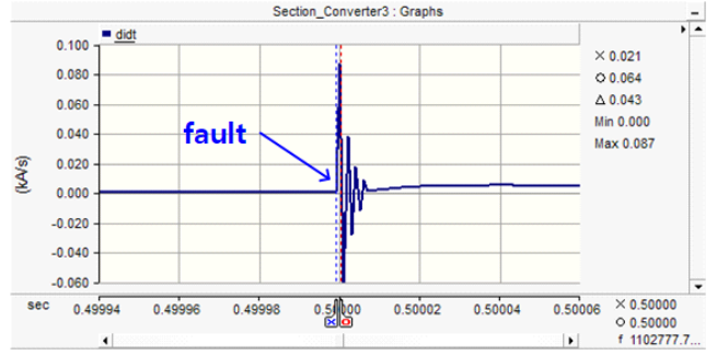
(c) 사고전류의 경사각 [그림 9] 사고전류의 경사각 특성
