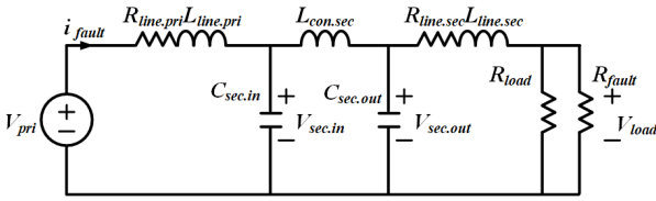
[그림 5] 단락사고 등가회로도
