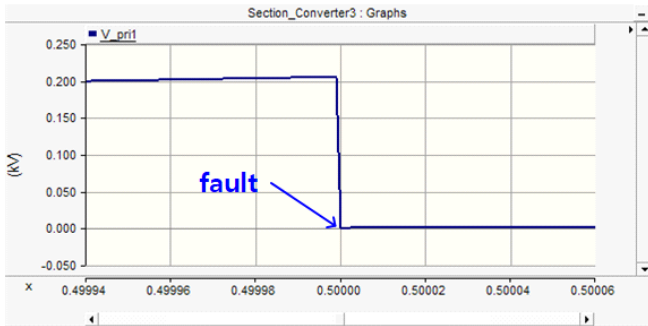
(a) 수용가전압
