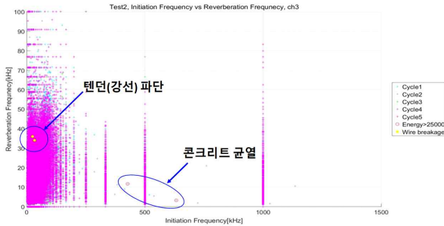
[그림 6] 텐던 파단 및 균열
