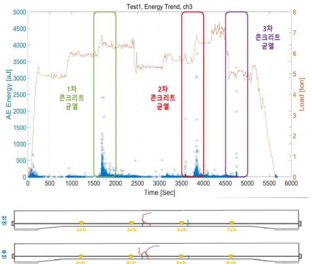
[그림 4] 철근콘크리트의 반복 하중시험
