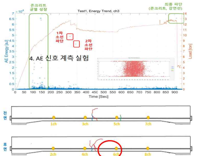
[그림 5] 철근콘크리트의 인장 파괴시험
