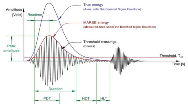
[그림 2] AE 아날로그 신호
