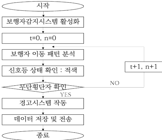
[그림 3] 보행자 무단횡단 시 차량경고 알고리즘
