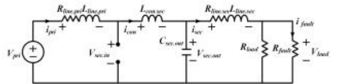
[그림 5] 단락사고 등가회로도
