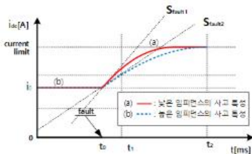
[그림 3] 구간컨버터의 임피던스에 따른 사고특성
